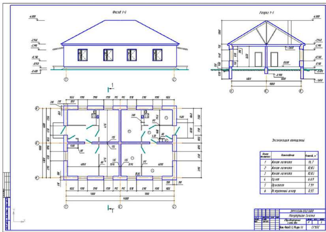
Будівельний кресленик одноповерхової споруди
