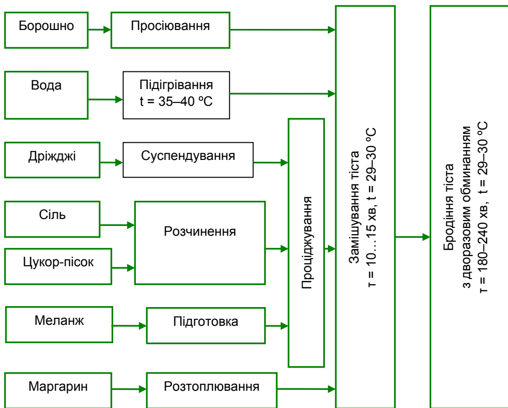
Технологічна схема приготування дріжджового безопарного тіста
