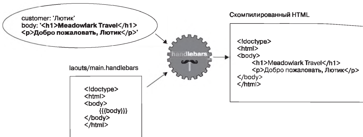
Рис. 7.2. Рендеринг представления с помощью макета
