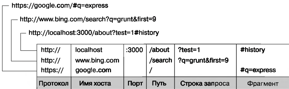
Рис. 6.1. URL и его составные части
