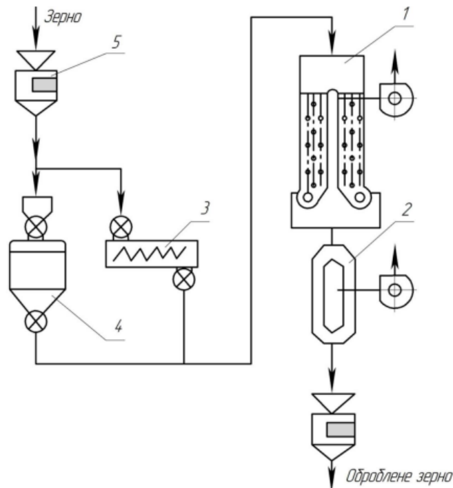
Рис.12.11 Технологічна схема гідротермічного оброблення зерна
