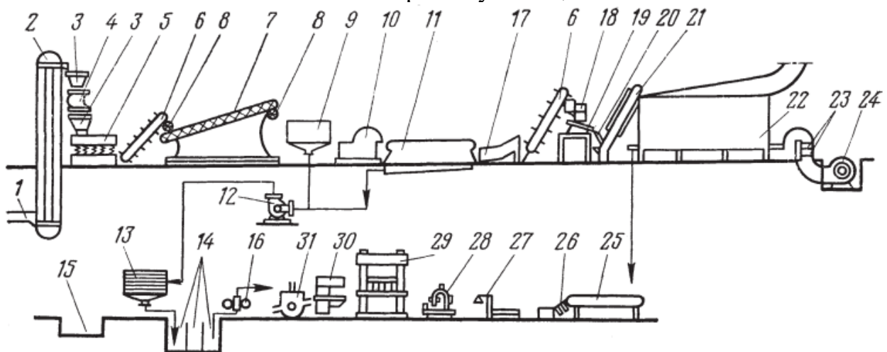
Рис.12.13 Апаратурно-технологічна схема приготування червоних столових виноматеріалів у потоці
