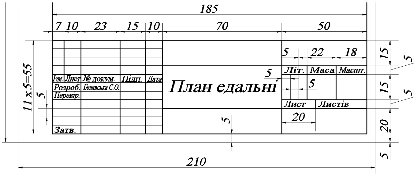
Рис.12.1.2 Основна напис і її розміри
