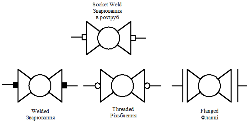
Рис.12.5 Схеми позначок затворів
