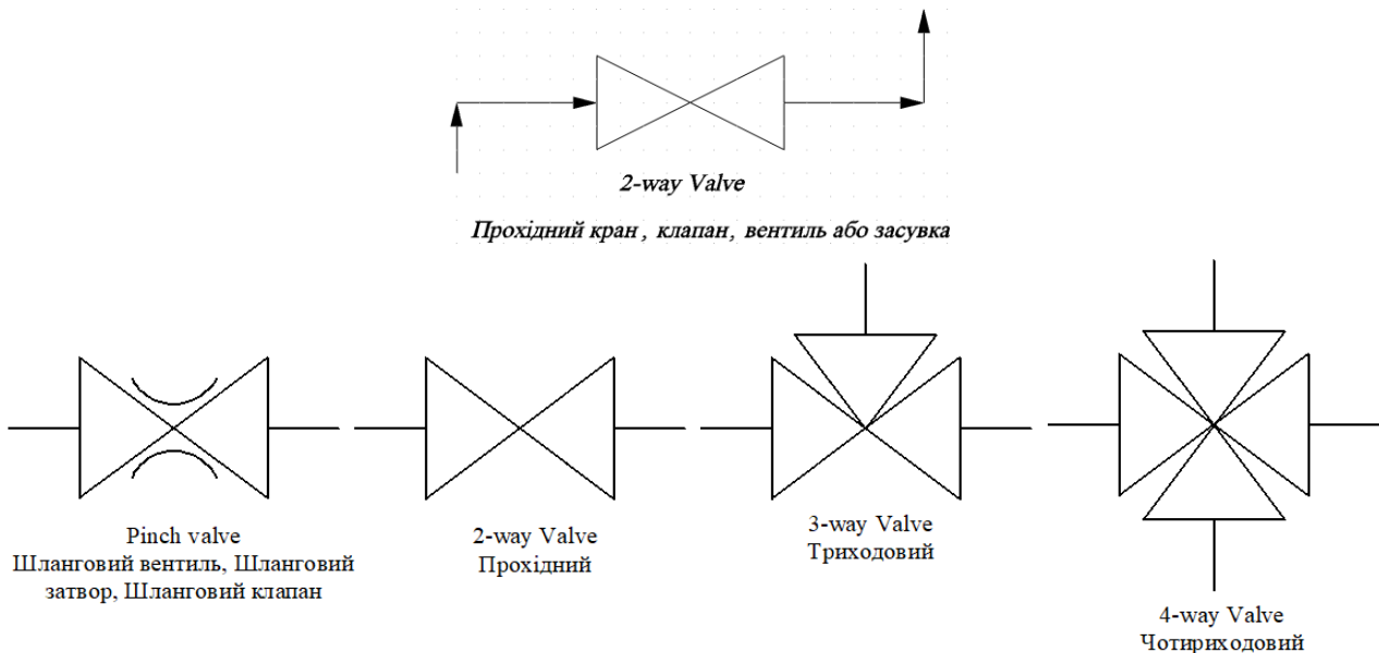
Рис.12.8 Схеми позначок кранів та вентелів
