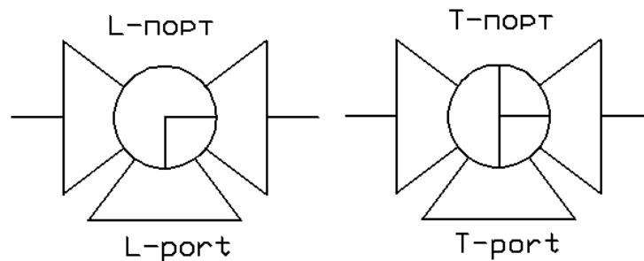
Рис.12.4 Схеми позначок для трьохходового крану
