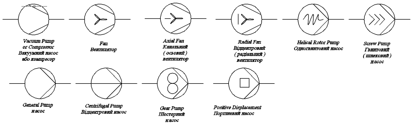
Рис.12.7 Схеми позначок насосів та вентиляторів
