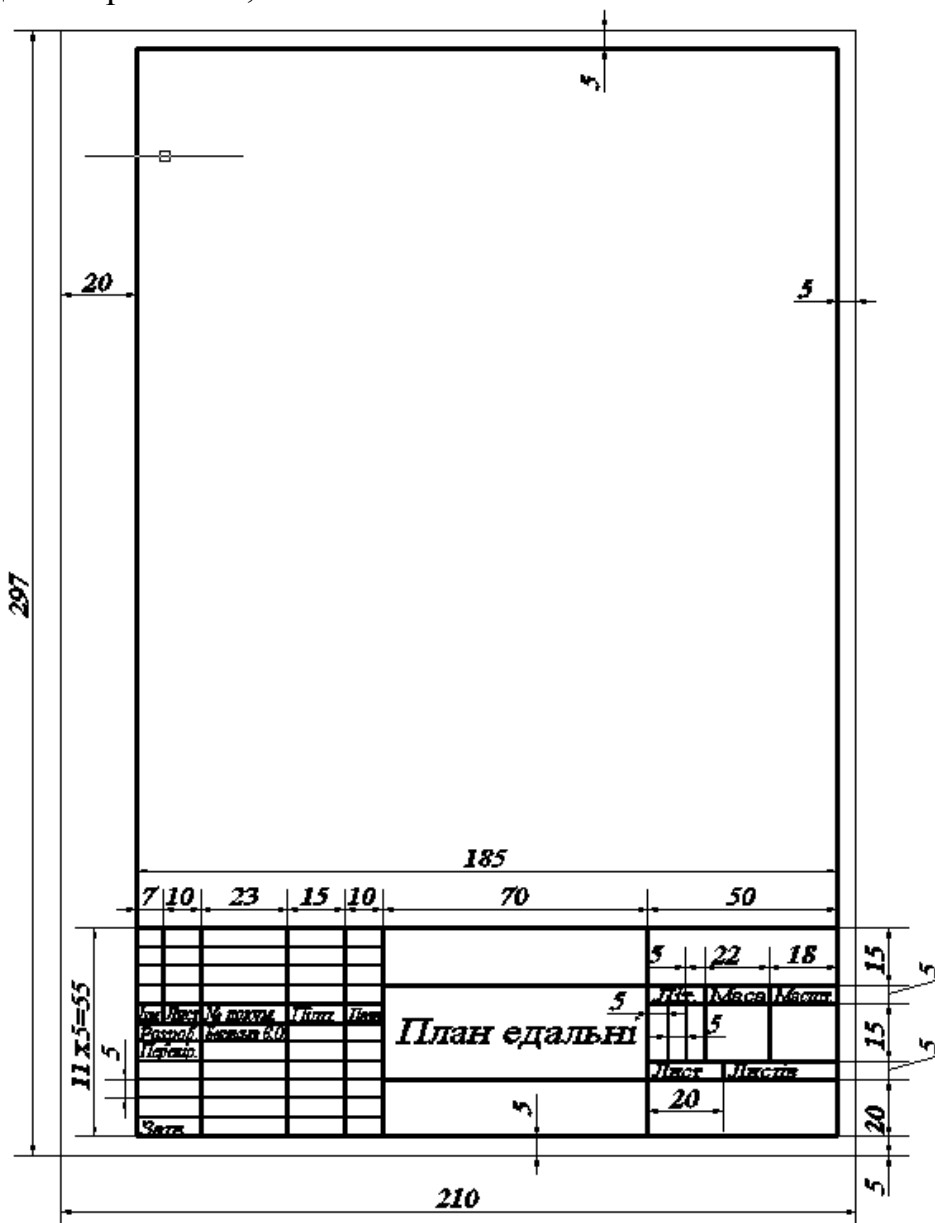
Рис.12.1.1 Оформлення поля креслення
