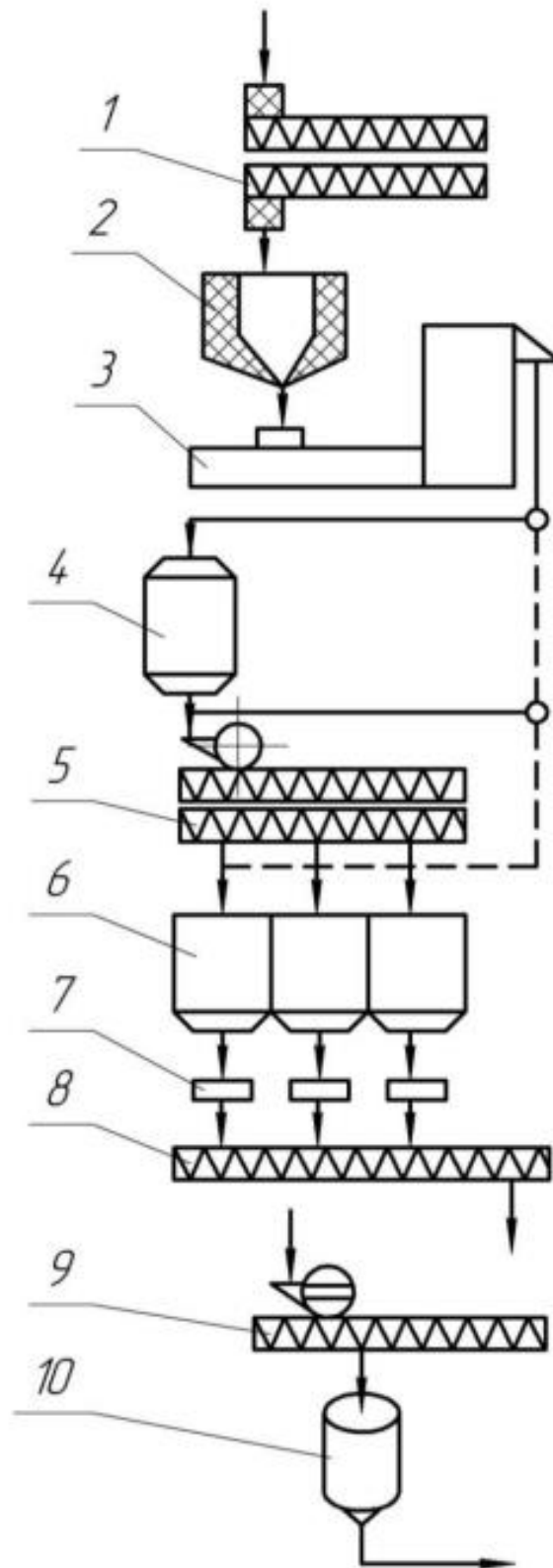
1 – апарат АШК; 2 – теплообмінник; 3 – мийна машина; 4 – вологознімач; 5, 9 – зволожувальні машини; 6 – бункер для відволоження; 7 – дозатор; 8 – змішувач; 10 – бункер для відволоження
