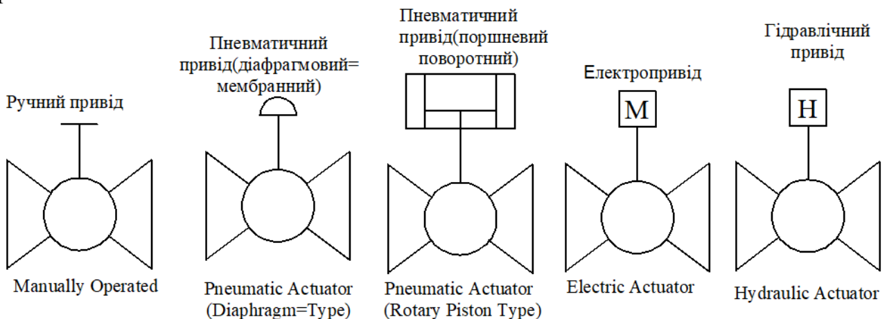
Рис.12.3 Схеми позначок приводів
