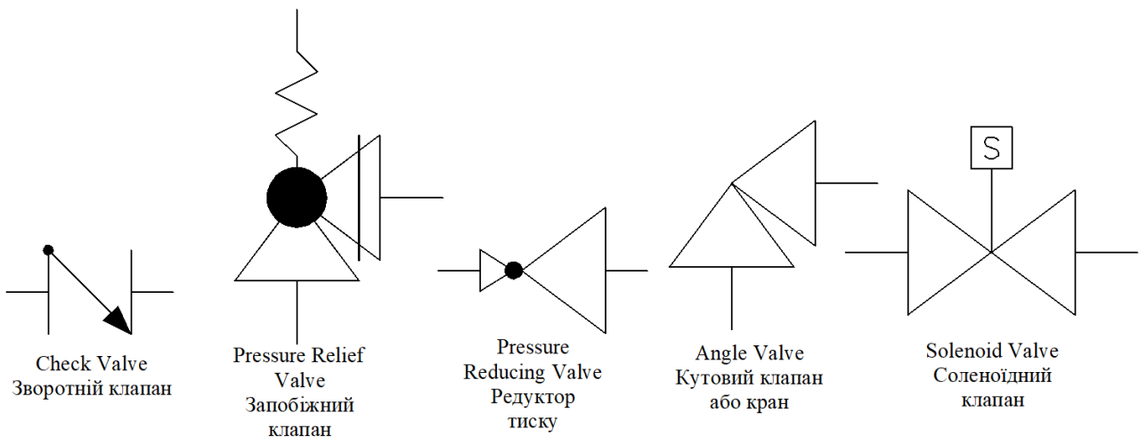
Рис.12.6 Схеми позначок клапанів
