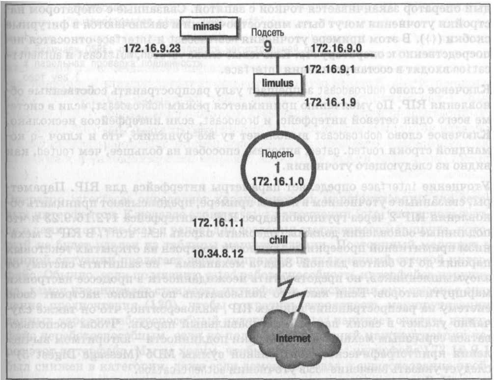
Рис. 7.4. Пример топологии маршрутизации
