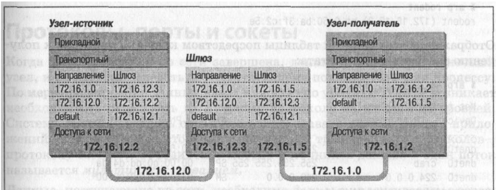
Рис. 2.4. Табличная маршрутизация
