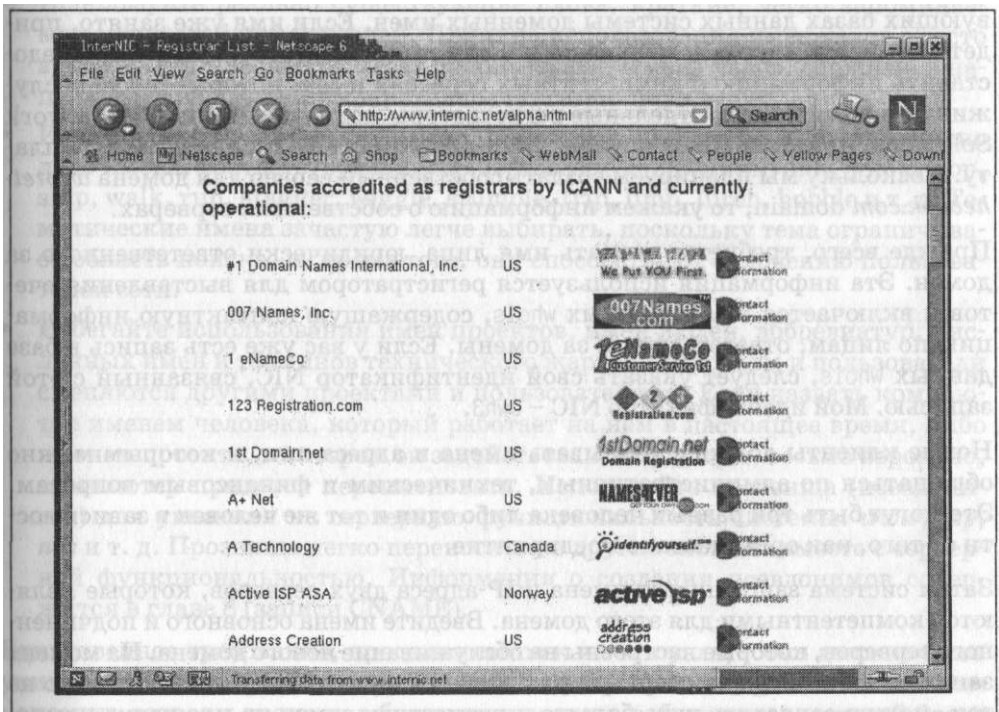
Рис. 4.2. Перечень регистраторов
