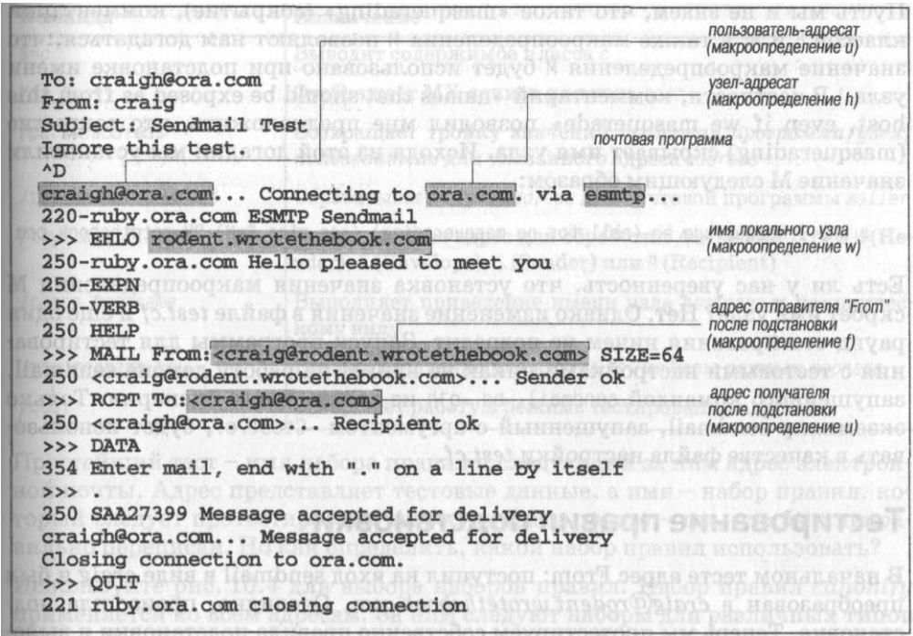
Рис. 10.5. Подробная диагностика
