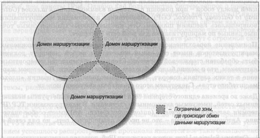
Рис. 2.3. Домены маршрутизации
