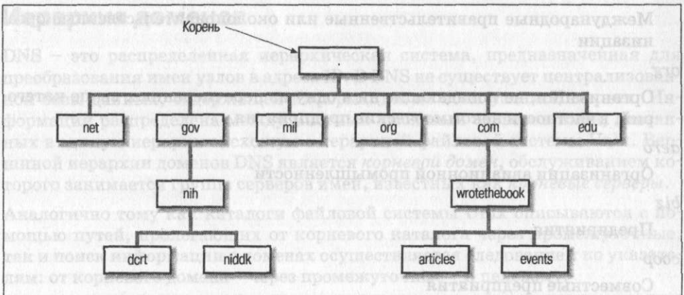
Рис. 3.1. Иерархия доменов
