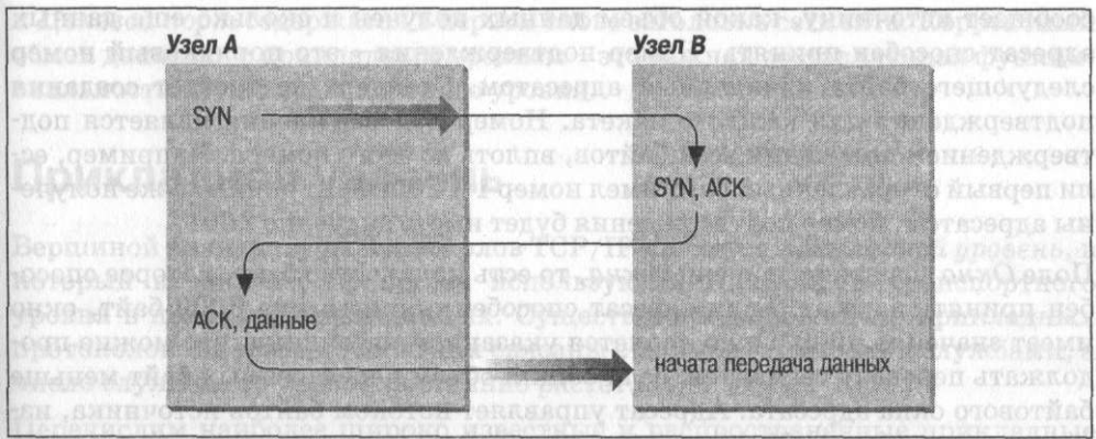
Рис. 1.10. Тройное рукопожатие
