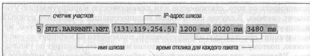
Рис. 13.2. Вывод traceroute
