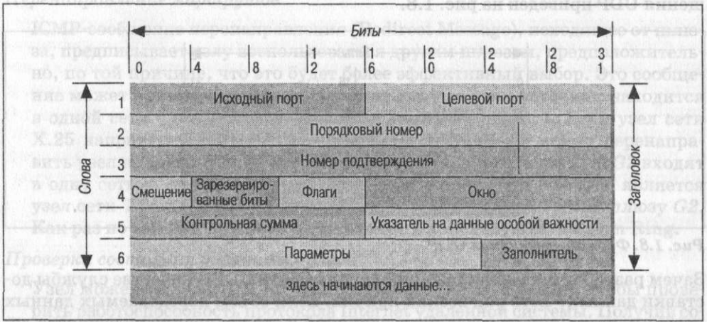
Рис. 1.9. Формат сегмента TCP
