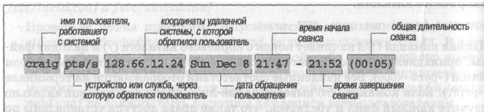
Рис. 12.3. Вывод команды last
