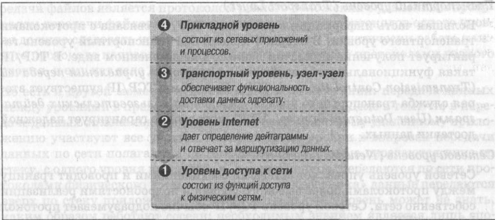
Рис. 1.2. Архитектура TCP/IP
