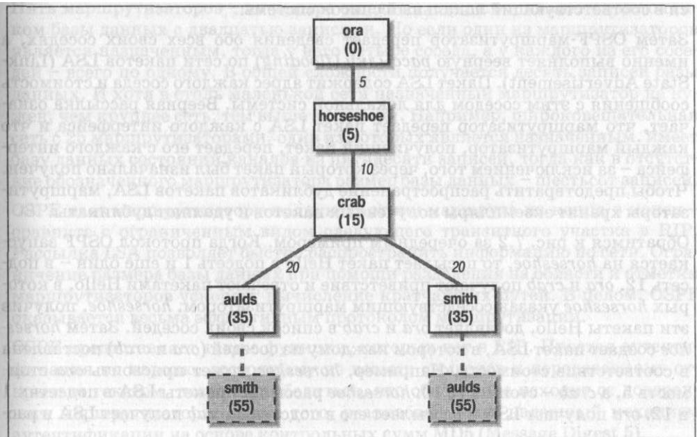
Рис. 7.3. Граф сети
