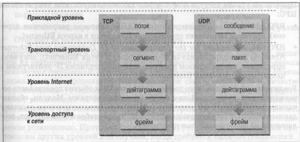
Рис. 1.4. Структуры данных
