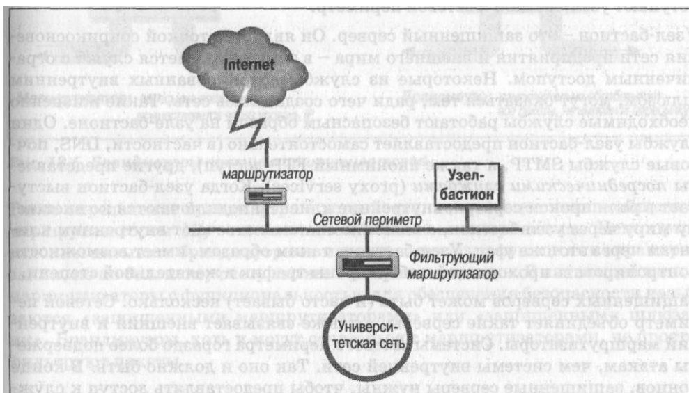
Рис. 12.4. Экранирование подсети
