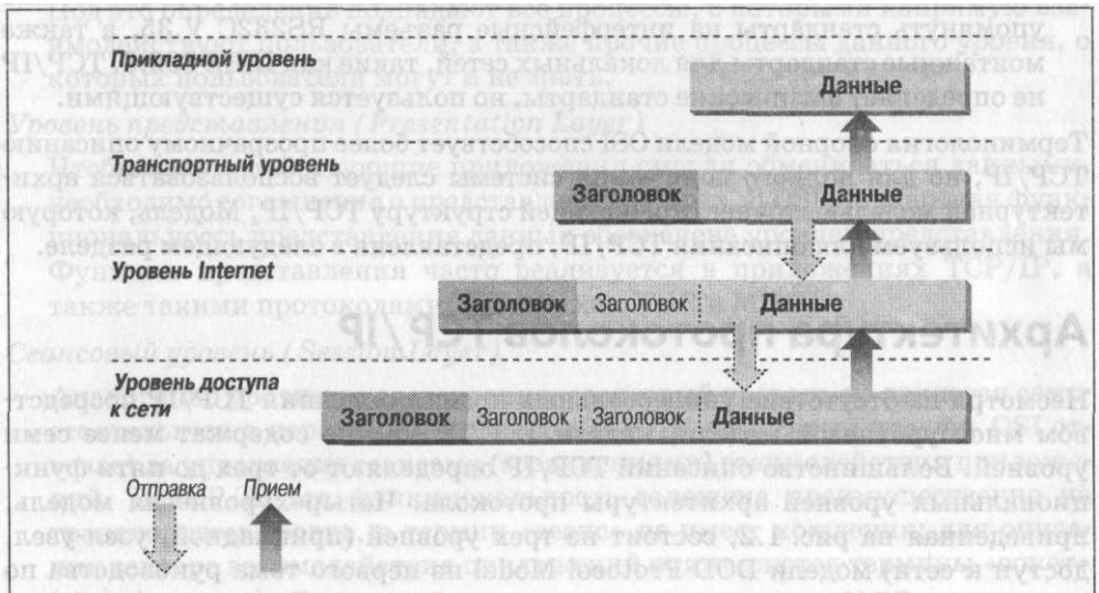
Рис. 1.3. Инкапсуляция данных
