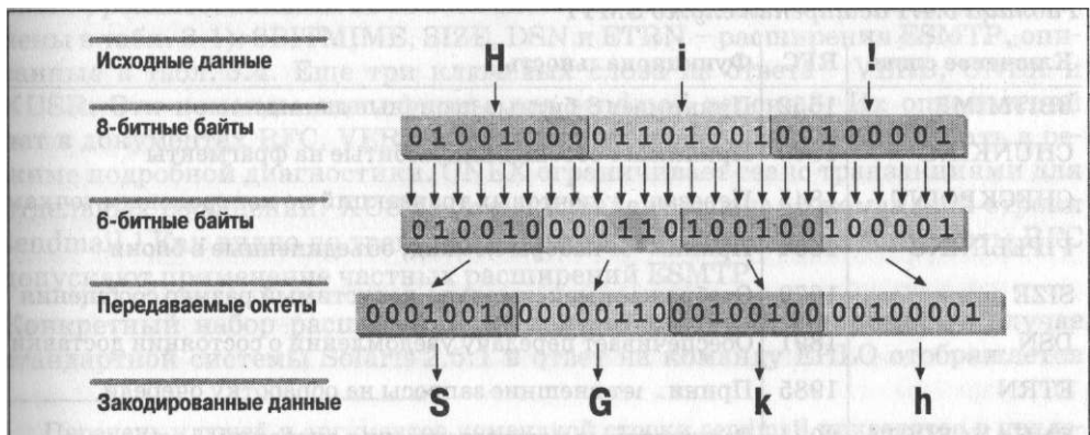
Рис. 3.4. Кодирование base64
