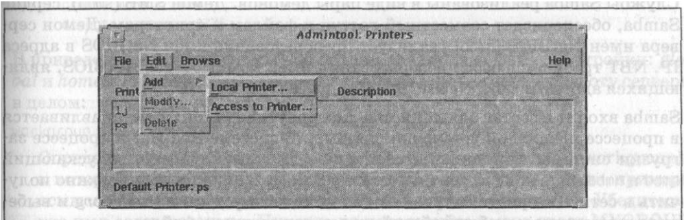
Рис. 9.1. Менеджер печати
