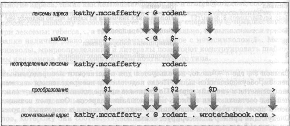
Рис. 10.3. Перетисывание адреса
