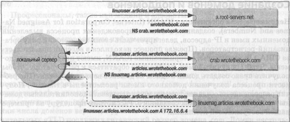
Рис. 3.2. DNS-запрос
