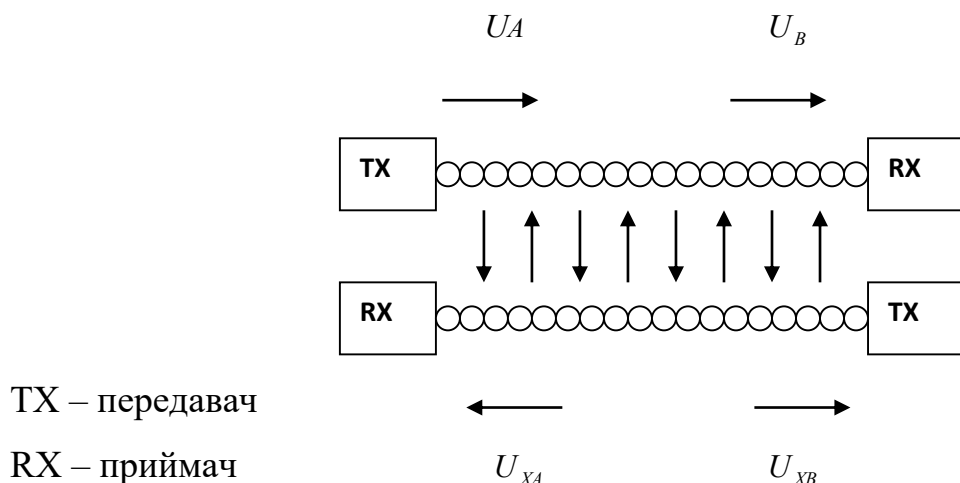
Рисунок 2.2 - Перехресні наведення
