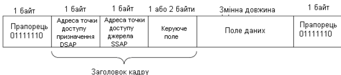
Рисунок 4.18 - Формат LLC-кадру
