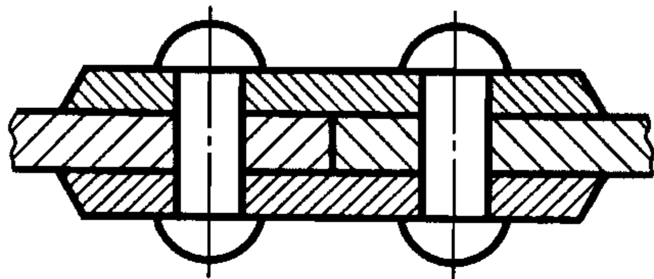
Черт. 10
