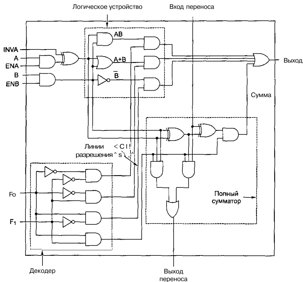
Рис. 3. 18. Одноразрядное АЛУ
