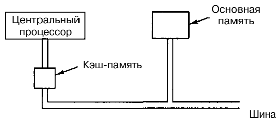
Рис. 2.13. Кэш-память по логике вещей должна находиться между процессором и основной памятью. В действительности существует три возможных варианта расположения кэш-памяти
