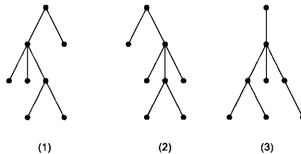
Рис. 9.8. Диаграммы деревьев
