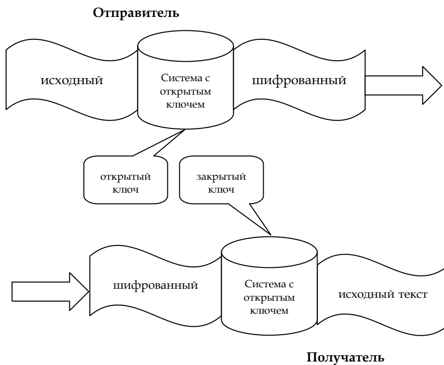
Рис. 6.4. Криптосистема с открытым ключом
