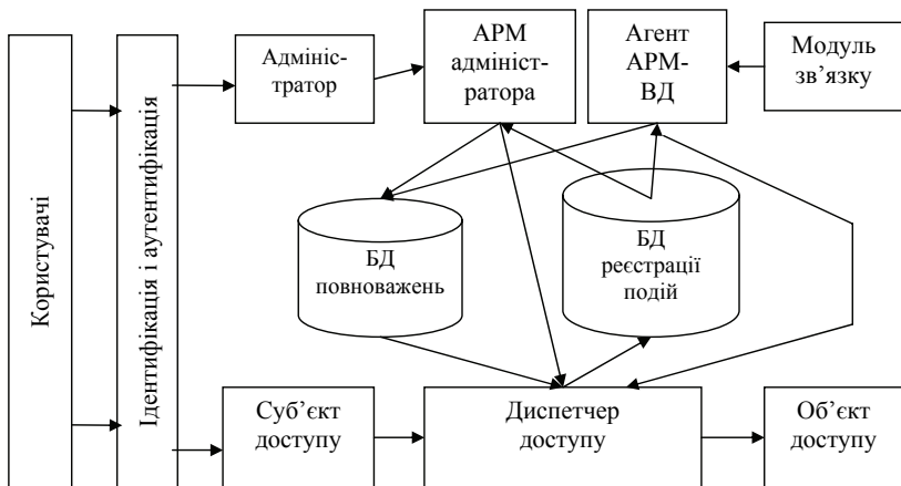
Рисунок 1.2 – Архітектура ПЗ КЗЗ на робочій станції
