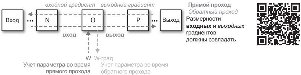
Рис. 3.2. ParamOperation с входом, выходом и параметрами
