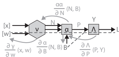
Рис. 2.5. Обратный проход по вычислительному графу линейной регрессии
