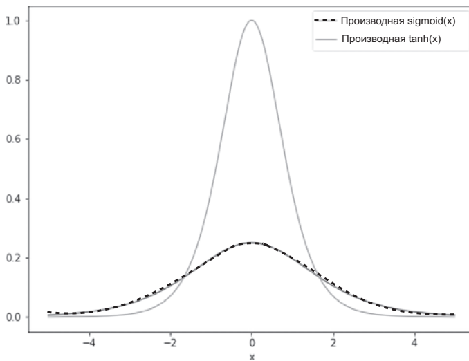
Рис. 4.7. Сигмоидная производная против производной tanh
