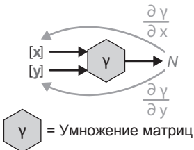
Рис. 1.17. Обратный проход операции умножения матриц
