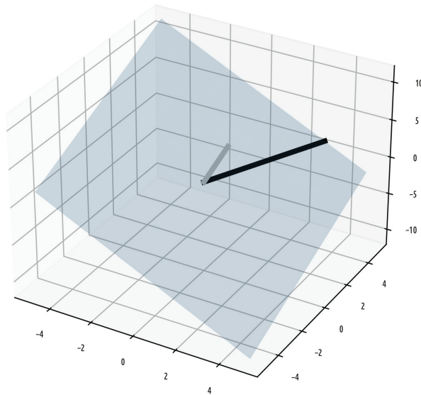
Рис. 6.3 ❖ Двумерное столбцовое пространство матрицы, встроеной в три измерения.
