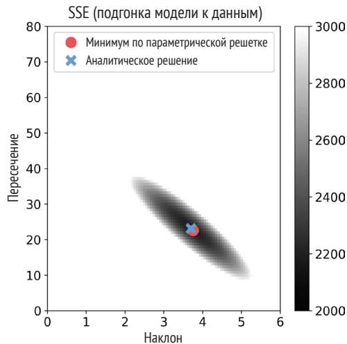
Рис. 12.8 ❖ Результаты поиска в параметрической решетке на наборе данных «Счастливого студента». Интенсивность показывает сумму квадратов ошибок, подогнанных к данным
