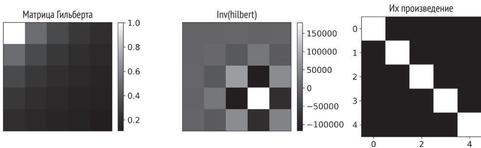
Рис. 8.5 ❖ Матрица Гильберта, обратная ей матрица и их произведение
