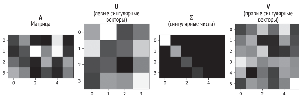
Рис. 14.2 ❖ Общая картина сингулярного разложения образцовой матрицы
