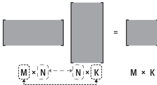
Рис. 5.3 ❖ Визуализация допустимости умножения матриц. Запомните эту картинку
