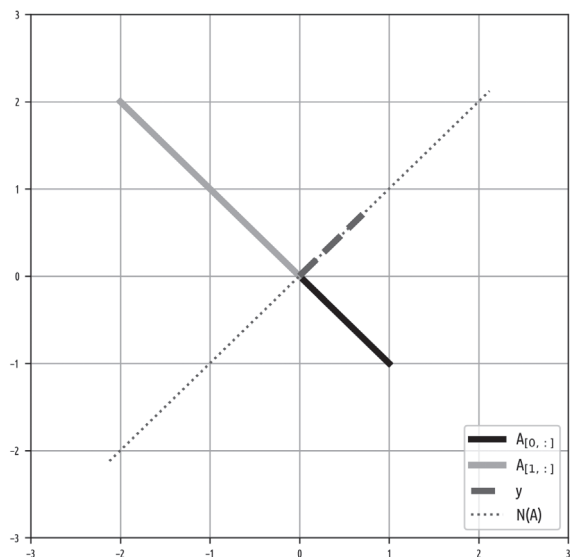
Рис. 6.4 ❖ Визуализация нуль-пространства матрицы
