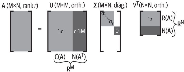
Рис. 14.1 ❖ Общая картина сингулярного разложения
