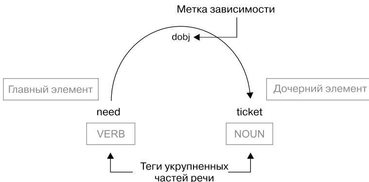
Рис. 2.3. Графическое представление дуги синтаксической зависимости
