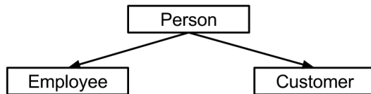
Рис. 27.2. Иерархия классов
