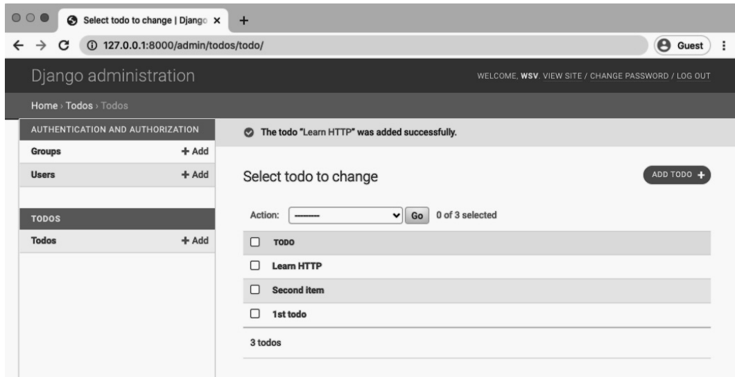
Admin todos
