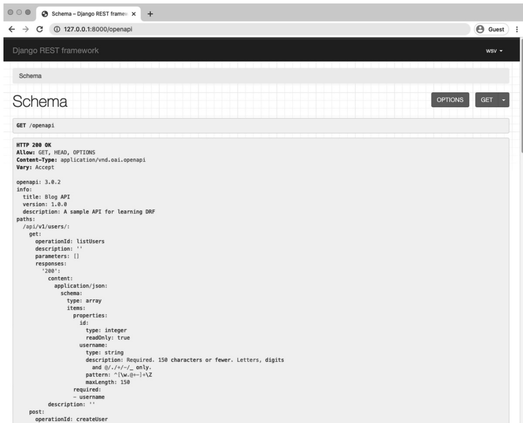
API Schema
