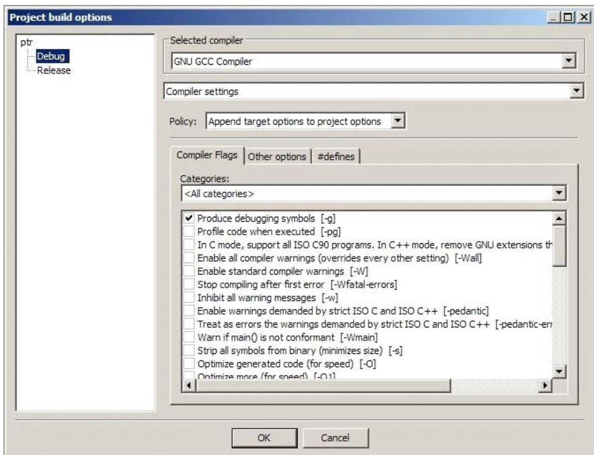
Рис. 20. Вікно налаштувань компіляції «Project build options»
