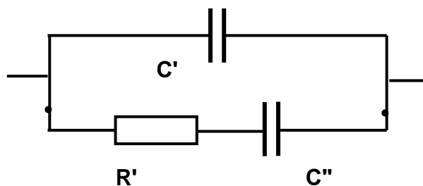
Рис. 3.11. Еквівалентна схема для моделювання абсорбції
