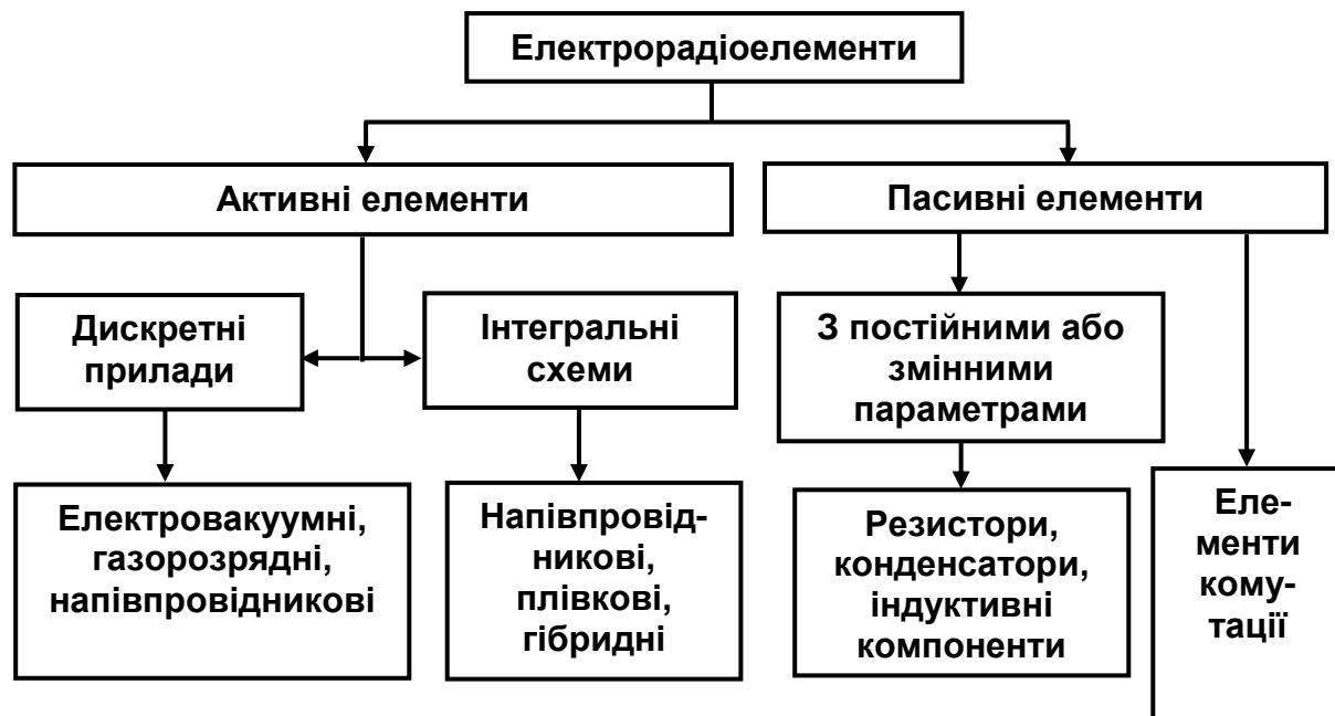
Рис. 1.1. Класифікація електрорадіоелементів
