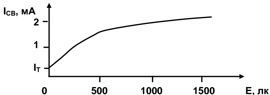
Рис. 2.9. Люкс-амперна характеристика
