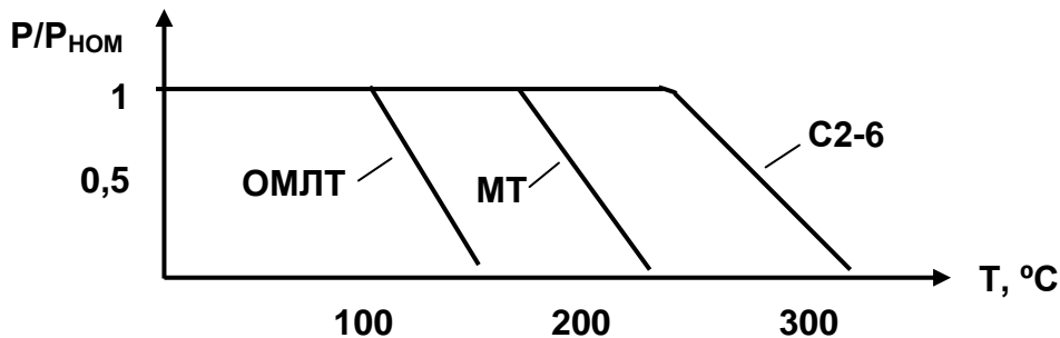
Рис. 2.3. Залежність потужності розсіювання від температури
