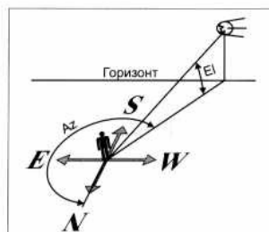
а) к определению азимута и угла места
