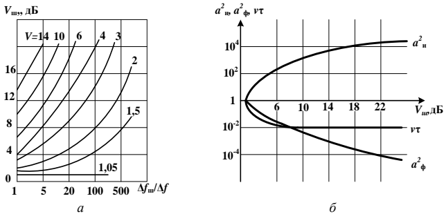
Рис. 7.3. Графік залежності значення амплітуди завади в РПП з широкою смугою від відношення \Delta f_w / \Delta f (а) та графік переходу від параметру V_{ш} до параметрів розподілу Вейбула (б)
