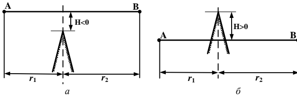
Рис. 6.9. Моделі радіотраси з клиновидною перепоною: a – виступ не затиноює лінії, що об’єднує антени в точках А і В; б – виступ затиноює лінію АВ
