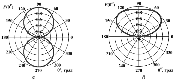
Рис. 5.3. Діаграми спрямованості диполя Надененко в площині E (а) та площині H (б) в полярній системі координат
