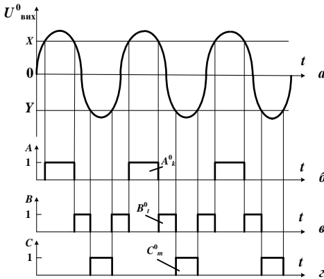
Рис. 7.5. Запис випробувального сигналу РПП: а – вихідна напруга генератора випробувальних сигналів; б – випадкові події стану A^0 ; в – випадкові події стану B^0 ; г – випадкові події стану C^0
