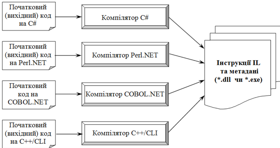
Рисунок 7.2. Всі .NET компілятори генерують інструкції IL та метадані
