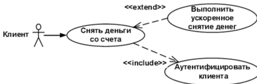
Рисунок 4.5. Приклад зв'язку включення й розширення
