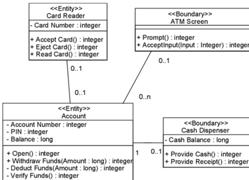
Рисунок 4.9. Приклад діаграми класів
