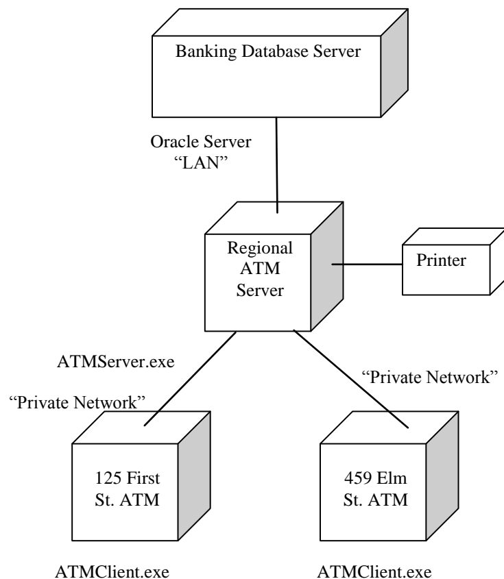
Рисунок 4.19. Приклад діаграми розміщення
