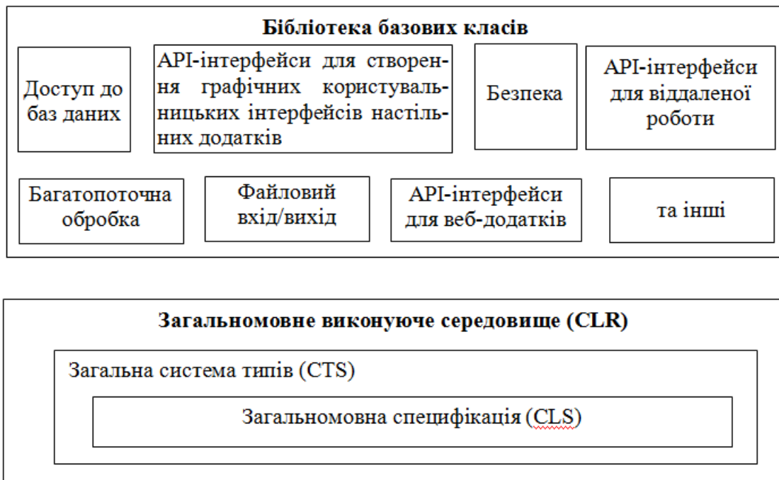
Рисунок 7.1. Відношення між CLR, CTS, CLS і бібліотеками базових класів
