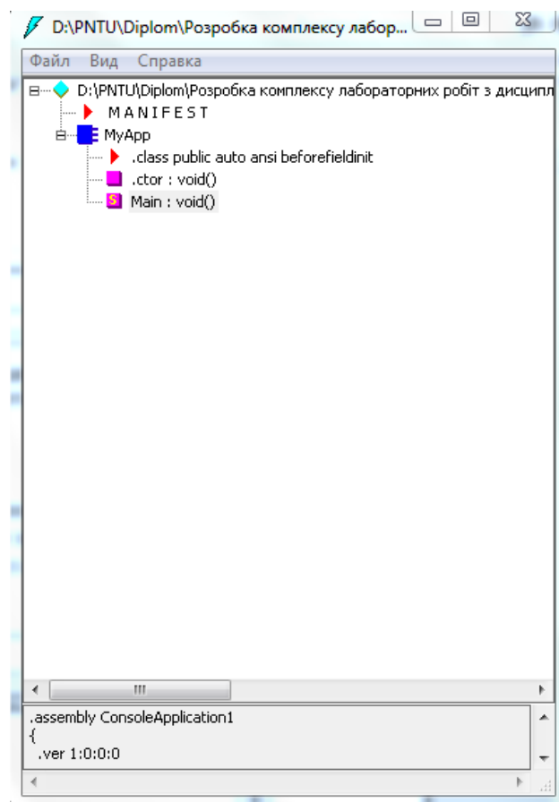
Рисунок 7.5. Утиліта ildasm.exe дозволяє бачити розміщені всередині збірки .NET код CIL, маніфест і метадані типів
