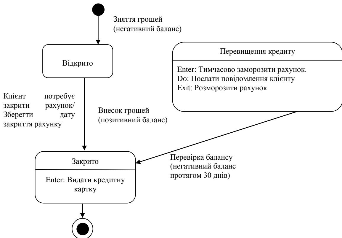
Рисунок 4.18. Приклад діаграми станів
