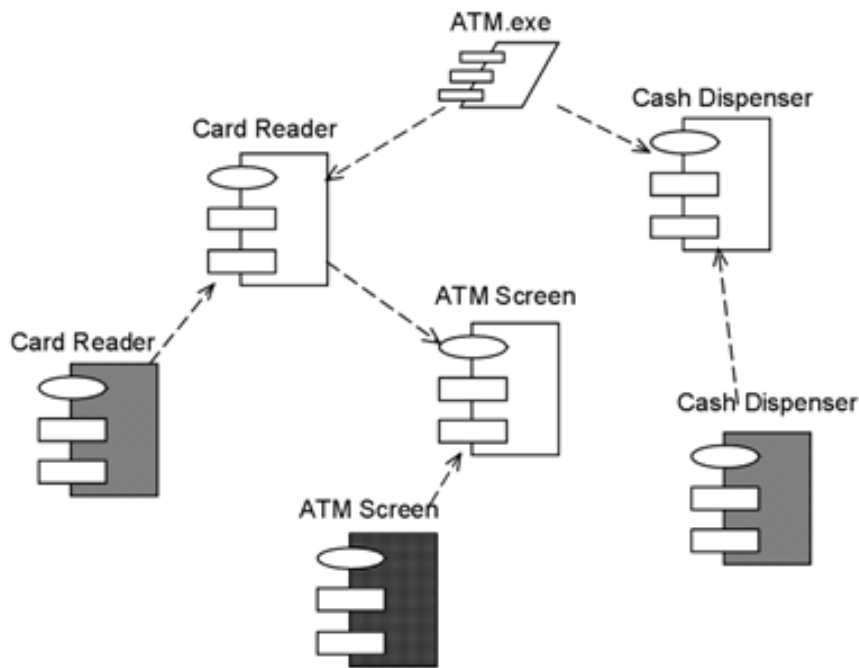
Рисунок 4.20. Приклад діаграми компонентів
