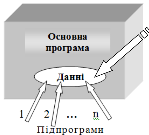
Рисунок 2.3. Архітектура програми з глобальною областю даних
