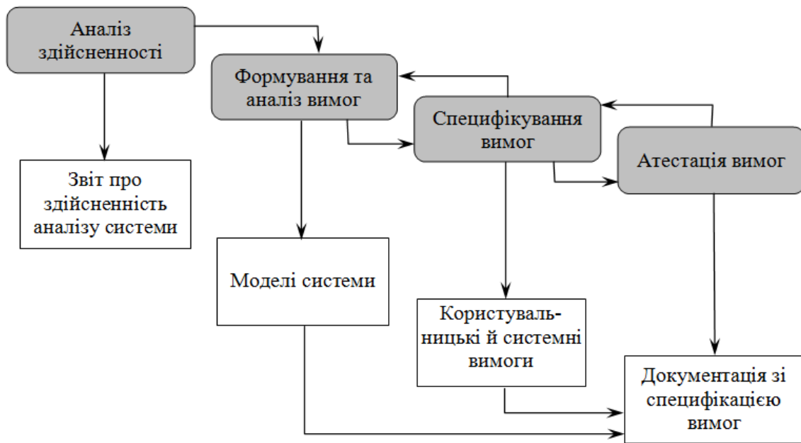
Рисунок 2.1. Процес розробки вимог
