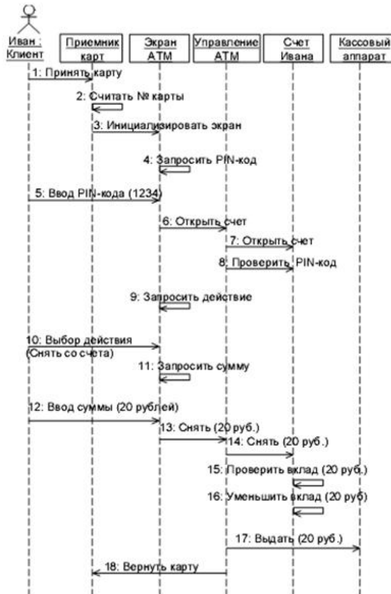
Рисунок 4.7. Пример диаграммы последовательности
