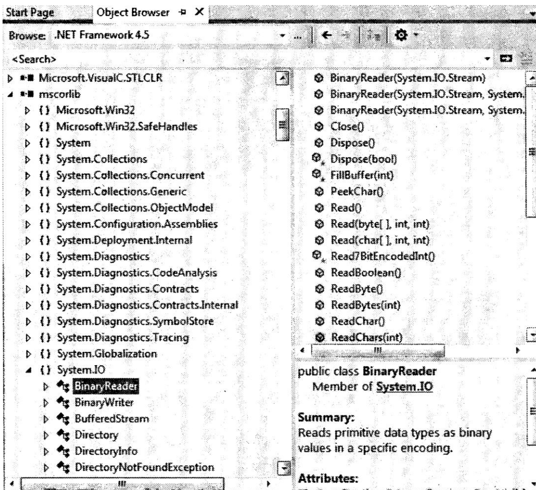
Рисунок 7.3. Збірка може мати будь-яку кількість просторів імен.
