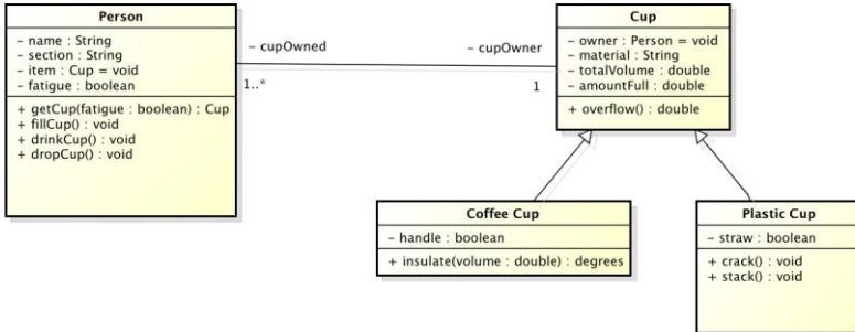
Рисунок 1.4. Діаграма класів
