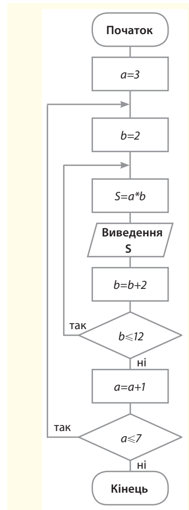
Рис. 15. Блок-схема алгоритму зі вкладеним циклом
