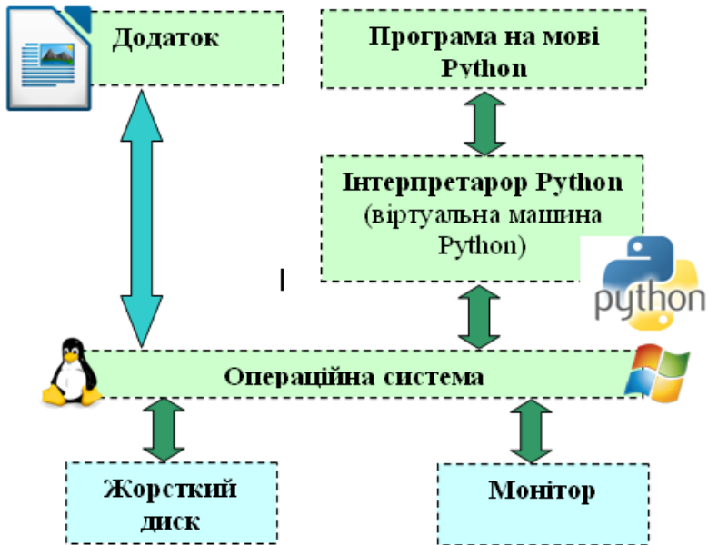
Рис. 2.1. Схема орієнтовної роботи програмі на мові Python
