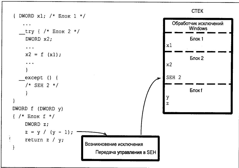
Рис. 4.1. SEH, блоки и функции
