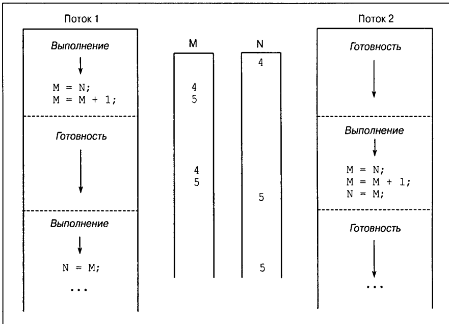
Рис. 8.1. Разделение общей памяти несинхронизированными потоками
