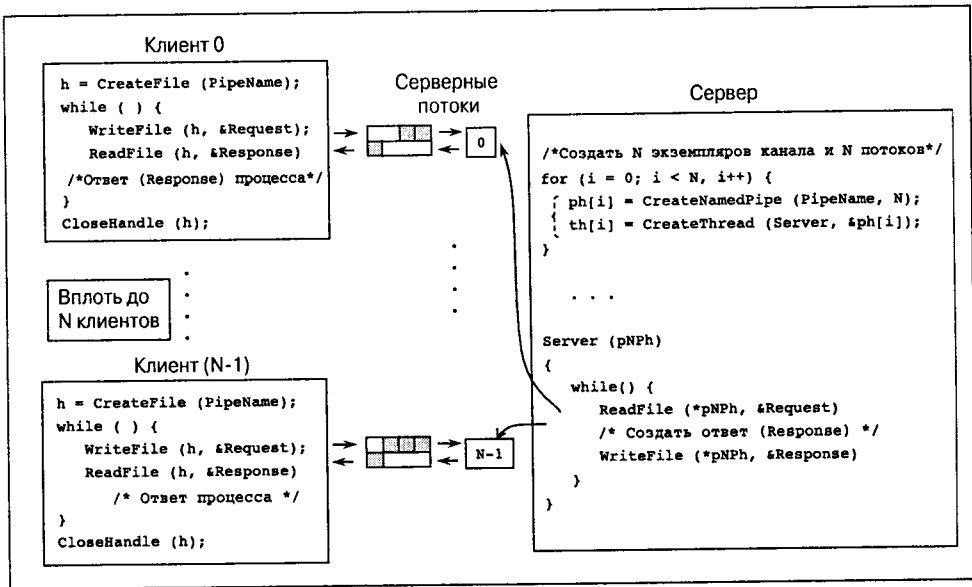
Рис. 11.2. Взаимодействие клиентов с сервером через именованные каналы
