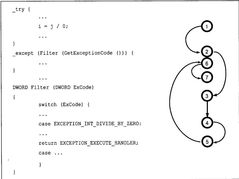
Рис. 4.2. Последовательность операций при обработке исключений
