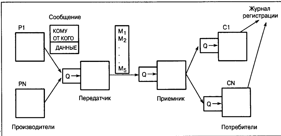
Рис. 10.1. Многоступенчатый конвейер
