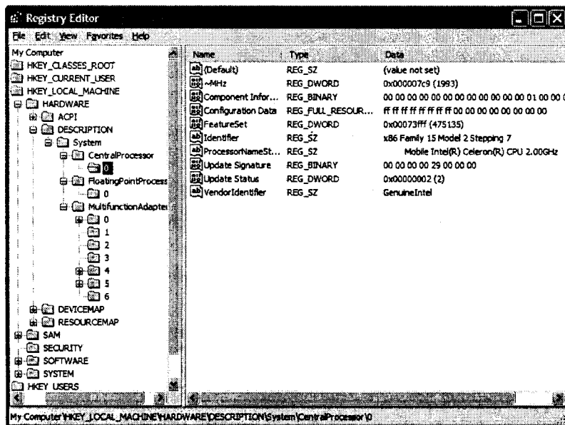
Рис. 3.1. Окно редактора реестра
