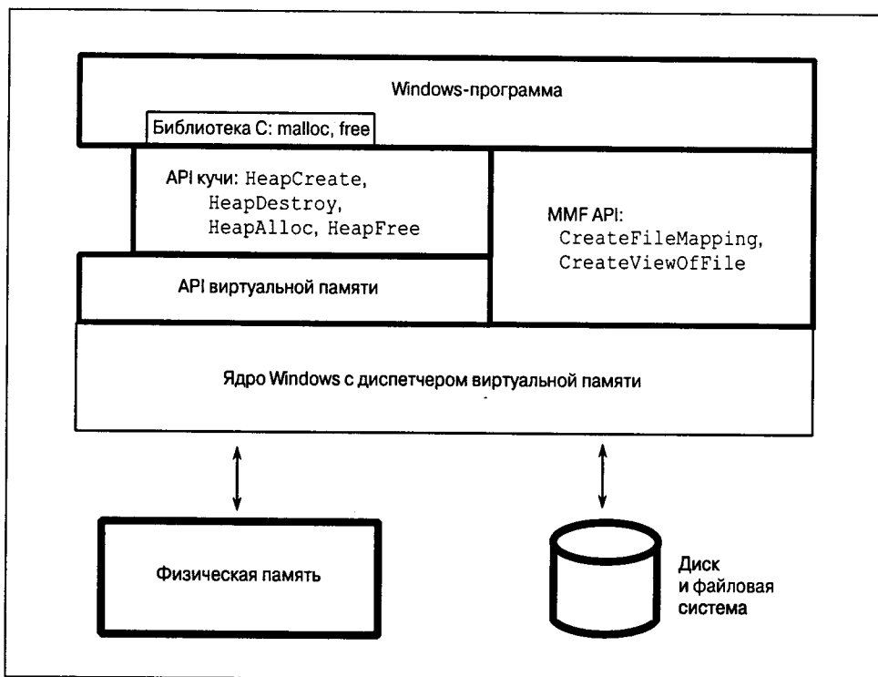
Рис. 5.1. Архитектура системы управления памятью Windows
