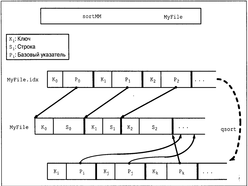
Рис. 5.5. Сортировка с использованием отображения индексного файла
