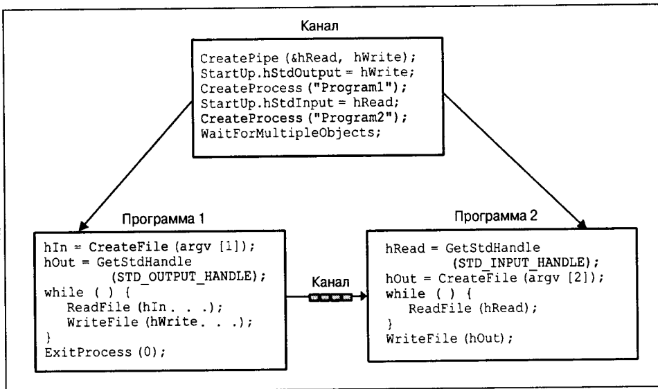
Рис. 11.1. Межпроцессное взаимодействие с использованием анонимного канала
