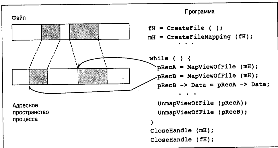
Рис. 5.3. Отображение представления файла на адресное пространство процесса
