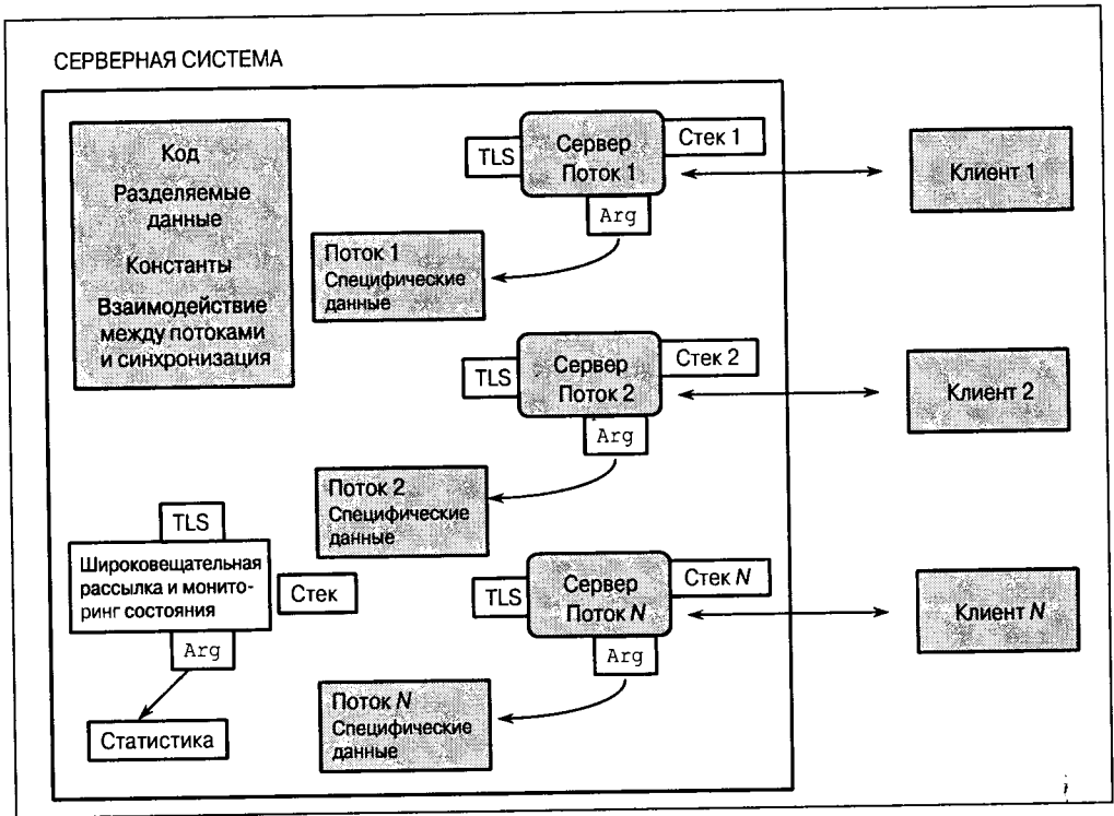
Рис. 7.1. Потоки в среде сервера
