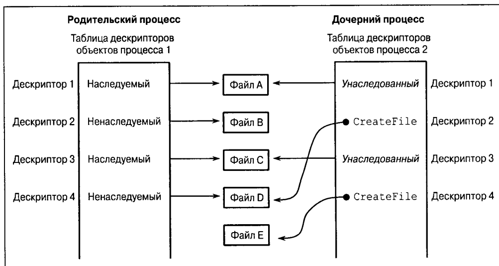
Рис. 6.2. Таблицы дескрипторов объектов для двух процессов
