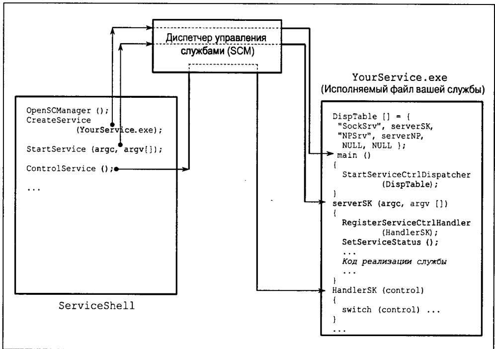
Рис. 13.1. Управление службами Windows через SCM
