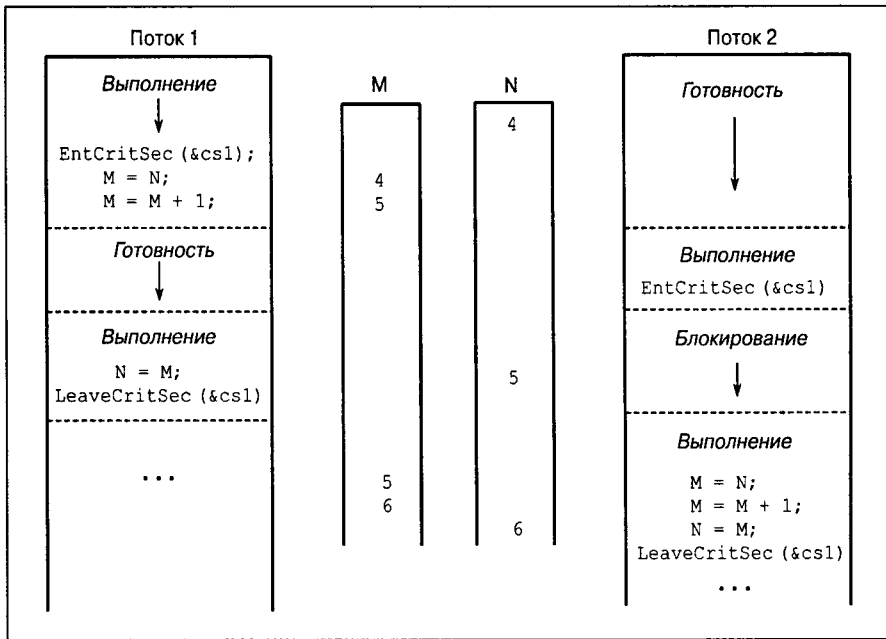
Рис. 8.2. Разделение общей памяти синхронизированными потоками
