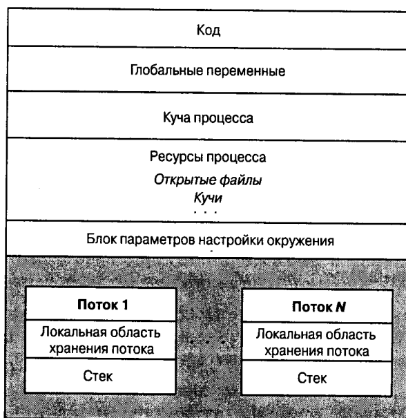
Рис. 6.1. Процесс и его потоки
