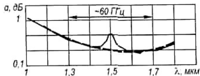
Рисунок 1.7 – Характеристика загасання оптичного волокна
