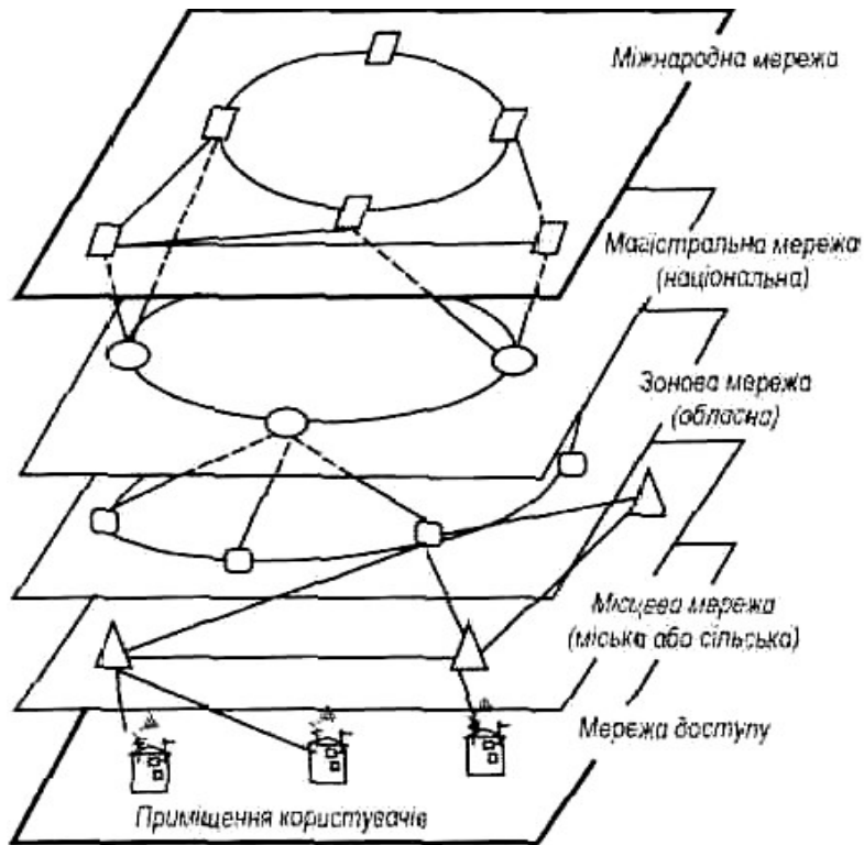
Рисунок 1.4 – Приклад побудови багаторівневої транспортної мережі
