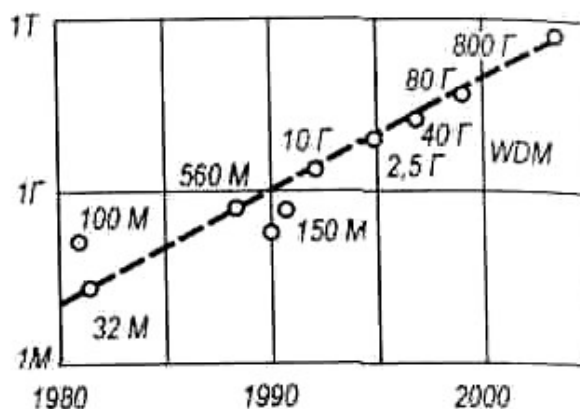
Рисунок 1.8 – Темпи освоєння пропускної здатності оптичного волокна протягом 1980-2003 рр. Значення пропускної здатності: М= 10^6 біт/с; Г= 10^9 біт/с, Т= 10^{12} біт/с; WDM – мультиплексування за довжиною хвилі
