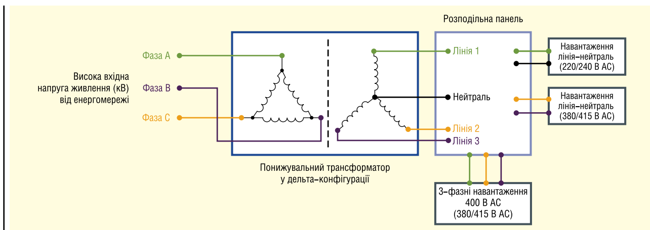
Рис. 3. Значення напруги типового європейського енергообладнання
