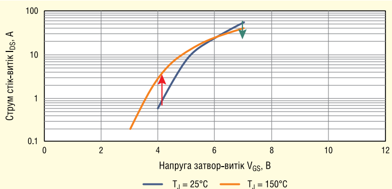
Рис. 2. Залежність напруги затвор–витік V_{GS} MOSFET від температури
