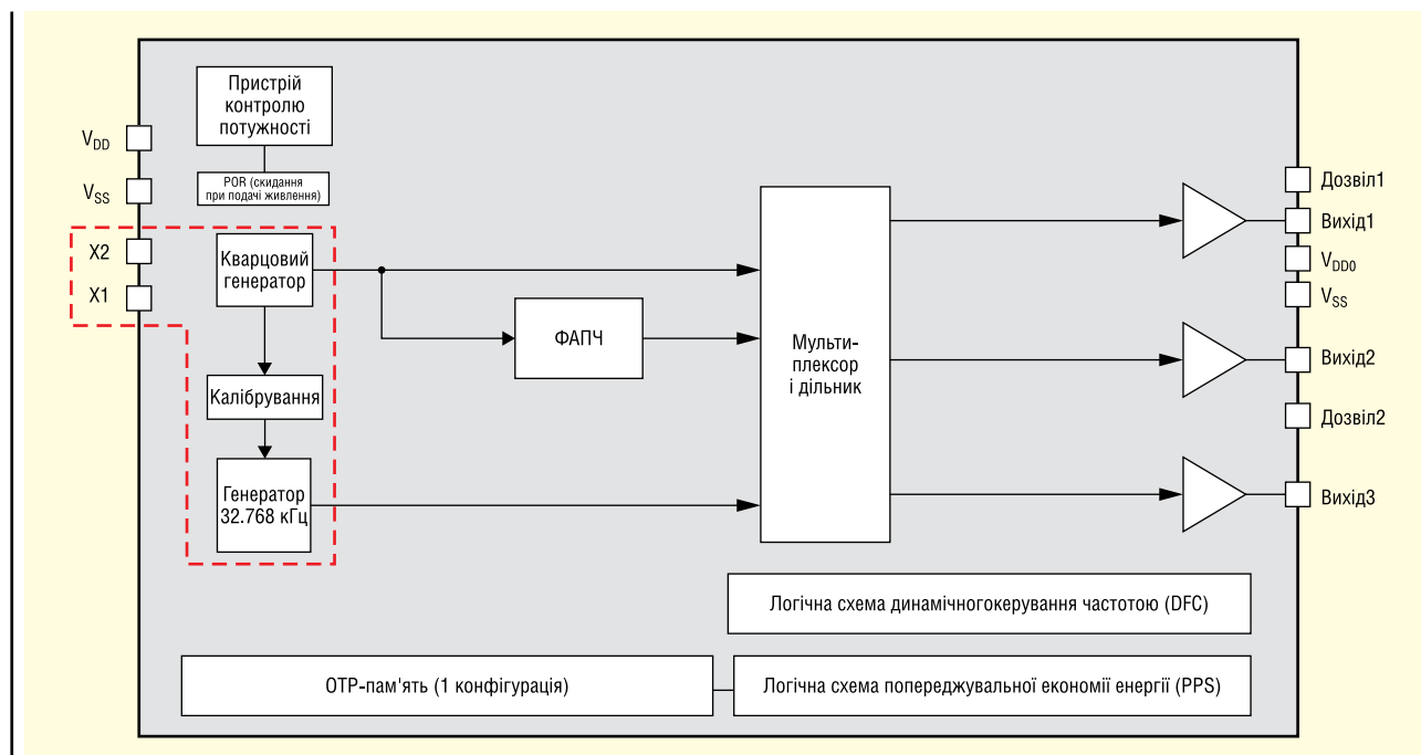
Рис. 1. Структурна схема пристрою MicroClock
