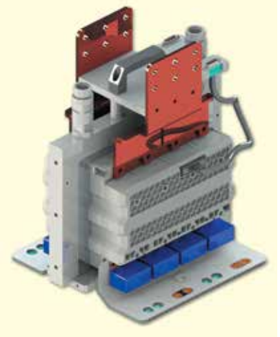
Рис. 7. Подвійний модуль SKiiP з охолоджувачем НРС
