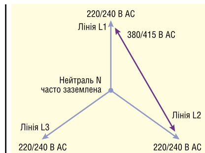
Рис. 2. Зіркоподібна конфігурація 380/415 В АС
