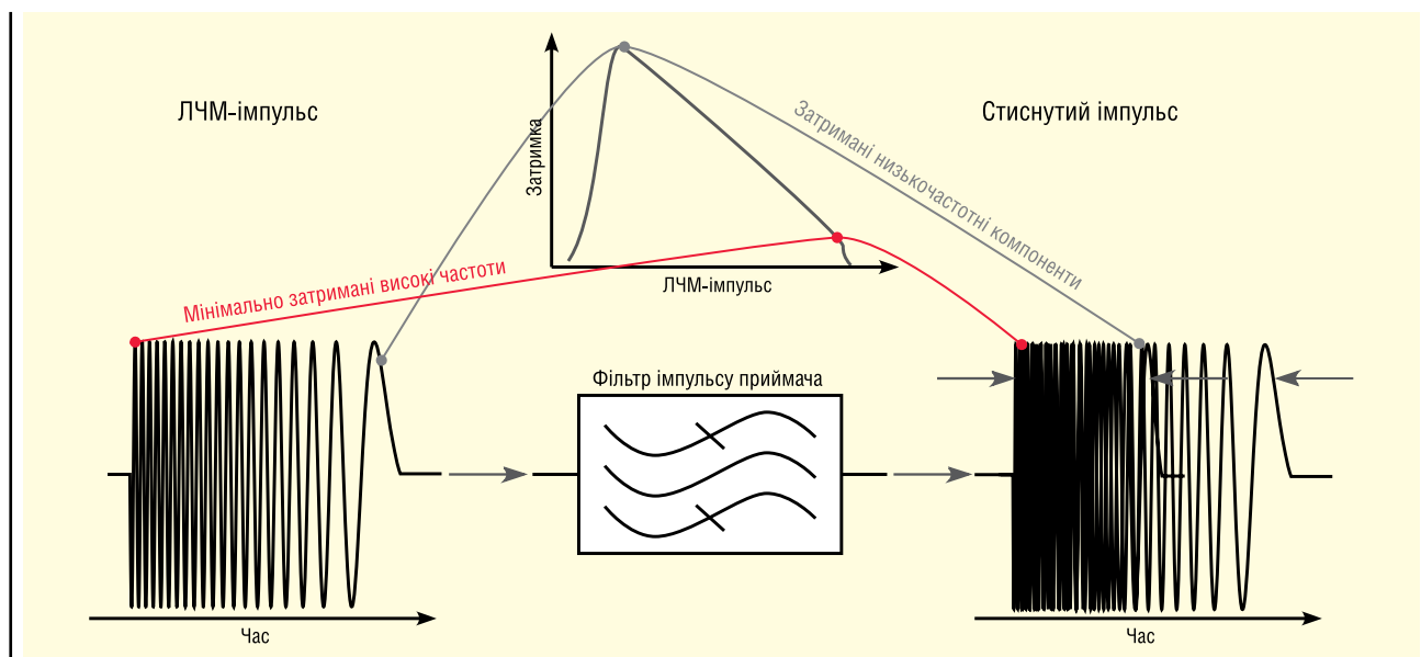
Рис. 2. Стиснення ЛЧМ імпульсу
