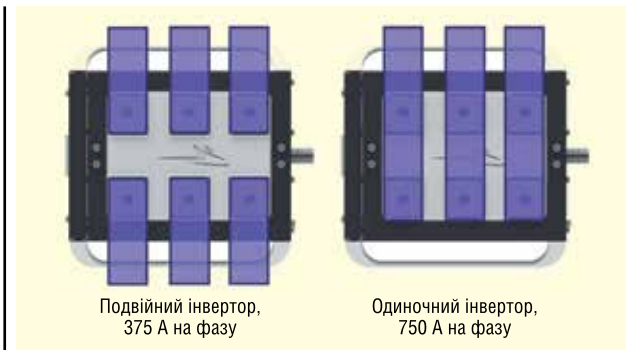
Рис. 7. Топологія вихідних шин забезпечує гнучкість для застосувань, що вимагають високого струму від одного інвертора
