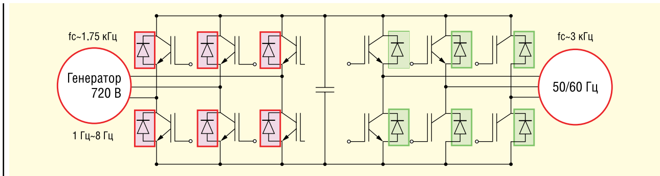
Рис. 4. Повномасштабна топологія back-to-back перетворювача
