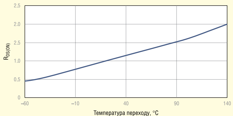
Рис. 1. У MOSFET — позитивний температурний коефіцієнт опору R_{DS(ON)}
