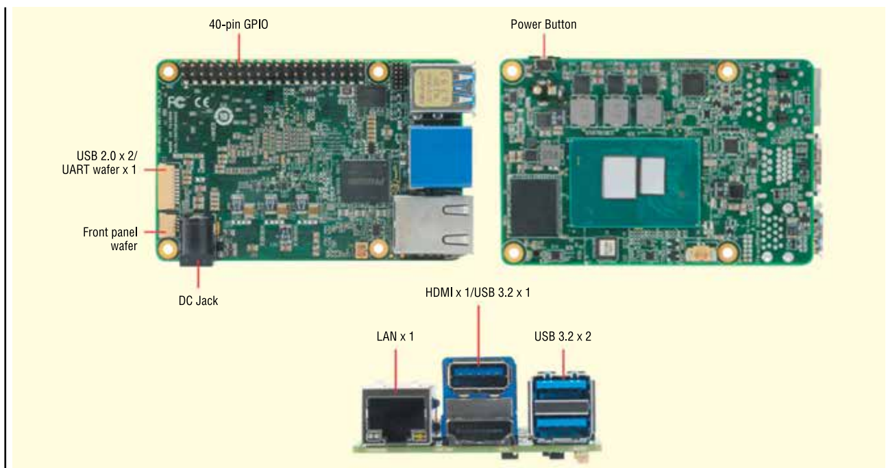
Рис. 1. Одноплатний комп'ютер AAEON UP 7000
