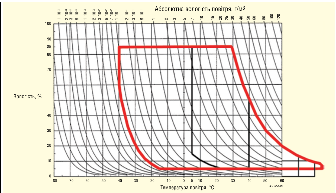
Рис. 3. Кліматичні умови класу 3К3 (чорний колір) і розширена область, досягнута SKiiP 4 (червоний колір)
