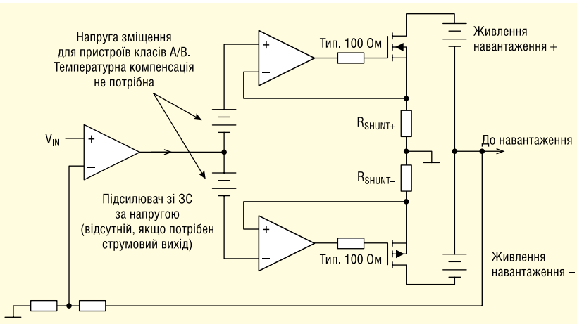
Рис. 5. У цій топології підсилювача потужності з лінійною вихідною напругою використовуються контури керування струмом для кожного MOSFET і загальний контур зворотного зв'язку за напругою
