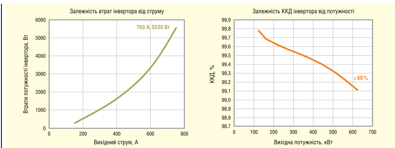
Рис. 8. Втрати потужності інвертора (ліворуч) і ККД (праворуч) за V_{dc} = 800 \text{ В} , f_{sw} = 10 \text{ кГц} , T_a = +25 \text{ °С}
