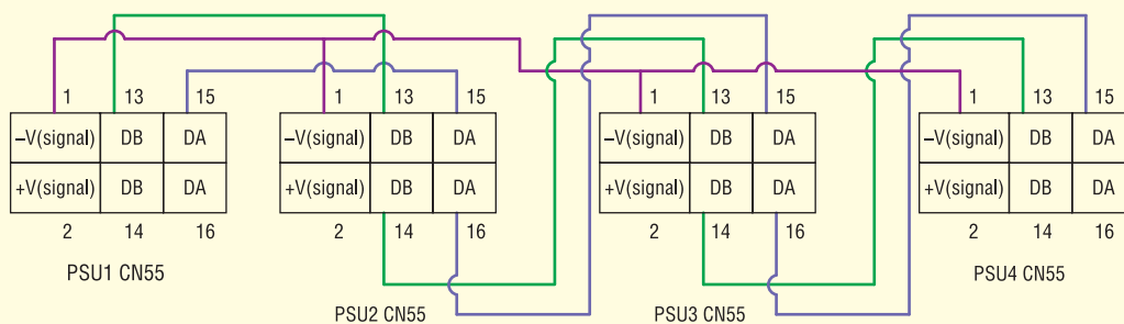
Рис. 33. Схема з'єднання контактів роз'ємів CN55 джерел живлення серії PHP-3500 у разі паралельного об'єднання чотирьох приладі
