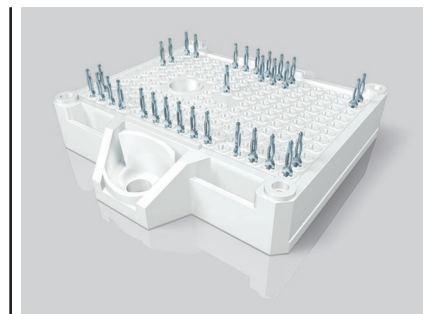
Рис. 2. SEMiTOP® E2, потужність до 120 кВт
