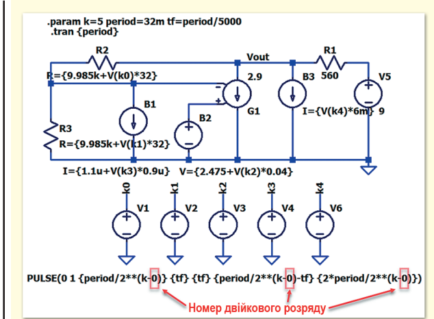
Рис. 3. Модель із генератором комбінацій на джерелах напруги
