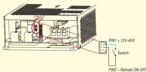
Рис. 31. Схема дистанційного ввімкнення/вимкнення джерел живлення сімейства PHP-3500
