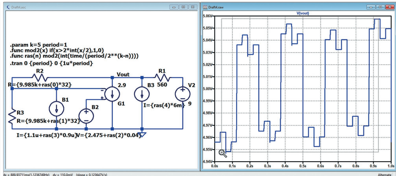
Рис. 6. Варіація параметрів за допомогою генератора двійкових комбінацій
