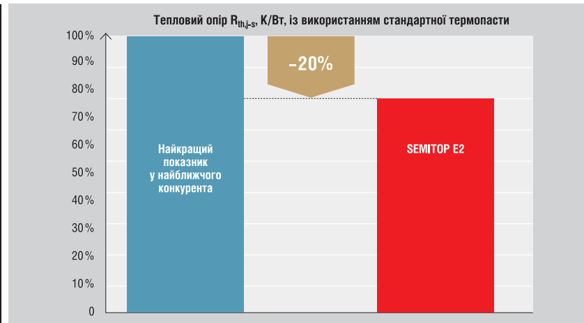
Рис. 4. При використанні стандартної термопасту тепловий опір модулів на основі SiC на 20% менший, ніж у найближчого конкурента
