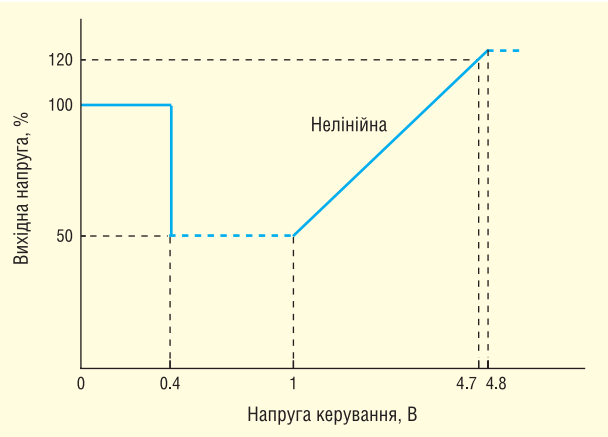
Рис. 25. Залежність вихідної напруги від напруги керування у джерел живлення серії PHP-3500
