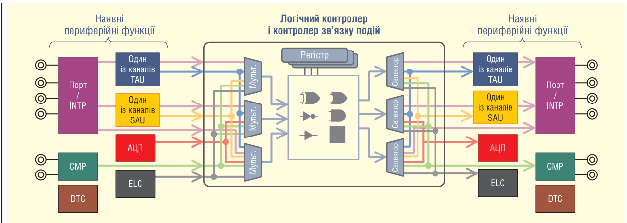
Рис. 7. Огляд контролера логіки та зв'язку подій
