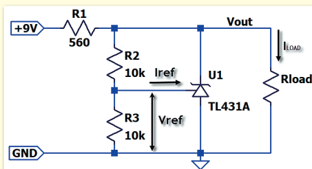
Рис. 1. Джерело опорної напруги
