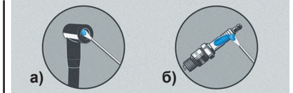
Рис. 2. Обережно нанесити мастило, намагаючись щоб воно не потрапило на клеми: всередину наконечника свічки запалювання (а); на керамічну поверхню свічки запалювання (б)
