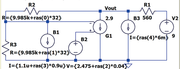
Рис. 5. Модель із генератором двійкових комбінацій
