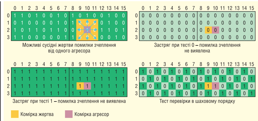
Рис. 1. Можливі помилки зчеплення між сусідніми бітами
