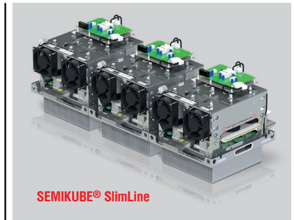
Рис. 5. Набір силових IGBT-модулів з повітряним охолодженням
