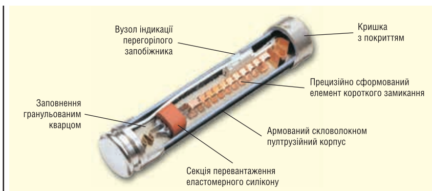
Рис. 9. Конструкція запобіжника LLSRK_ID
