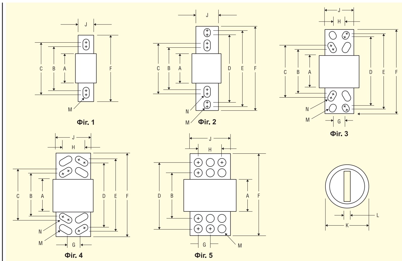
Рис. 2. Корпуси, у яких виготовляють запобіжники серії KLPC
