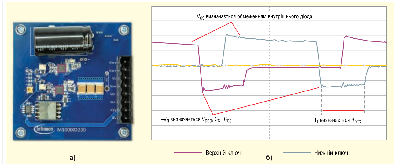
Рис. 7. Тестувальна плата розробника (а); осцилограми її роботи (б)
