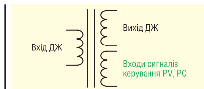
Рис. 2. Гальванічна ізоляція функцій PV, PC
