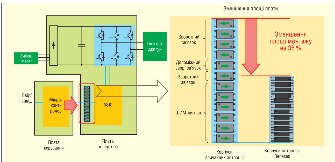
Рис. 2. Корпуси мікросхем серій RV1S92xxA і RV1S22xxA дають змогу заощадити до 35% займаної площі
