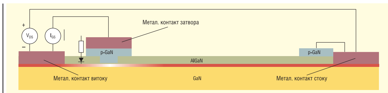
Рис. 1. Поперечний переріз силового ключа сімейства CoolGaN GIT
